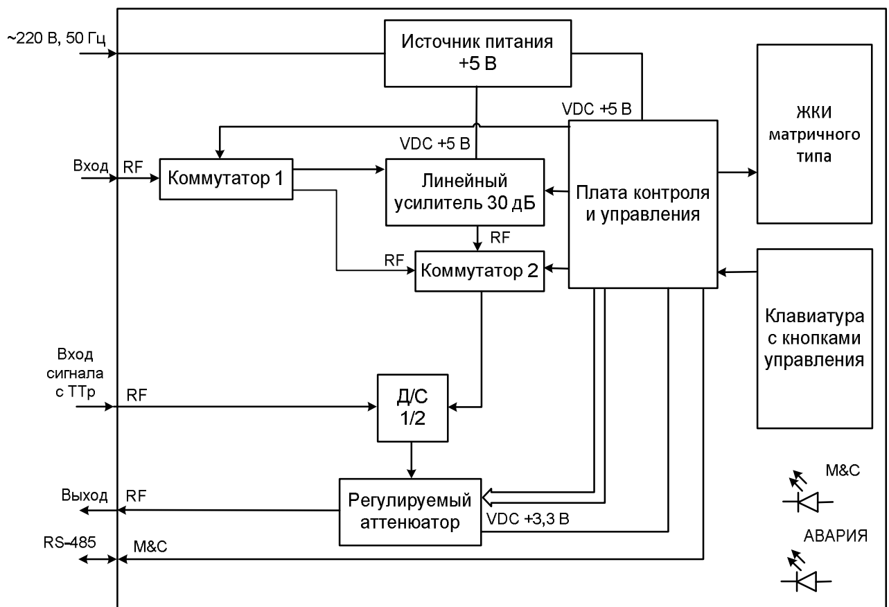
Рисунок 1.2 Функциональная схема ЛУА S
