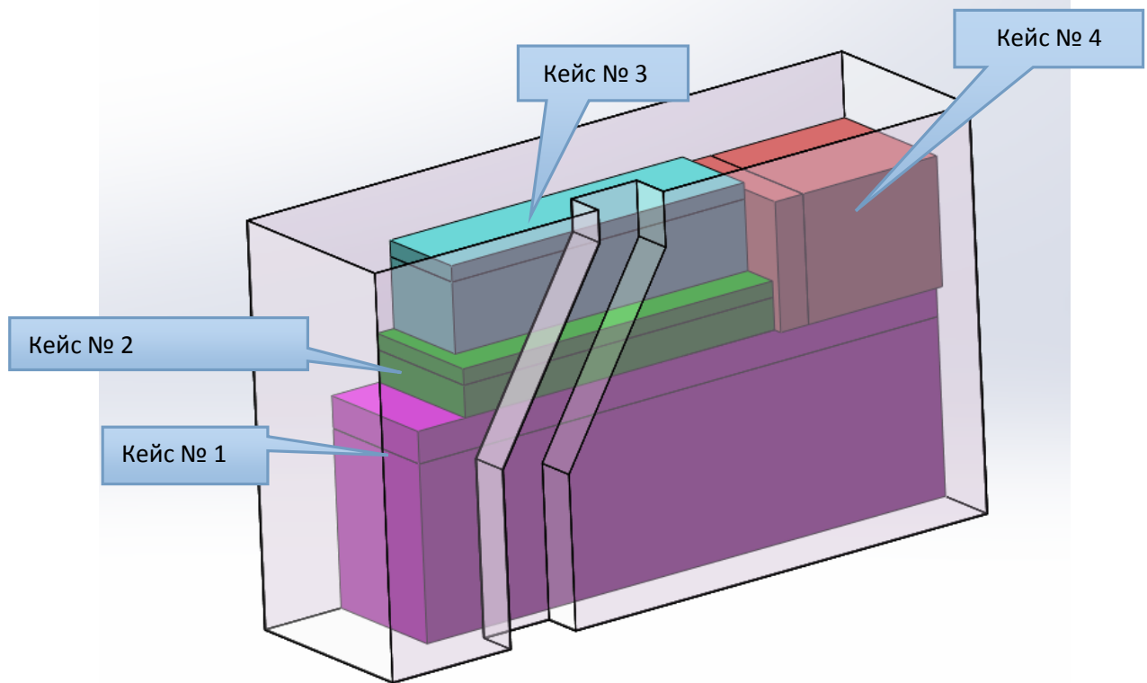
Рисунок 1.2.6 – Размещение кейсов АС 1.8 м Ки/С-диапазона при транспортировке
