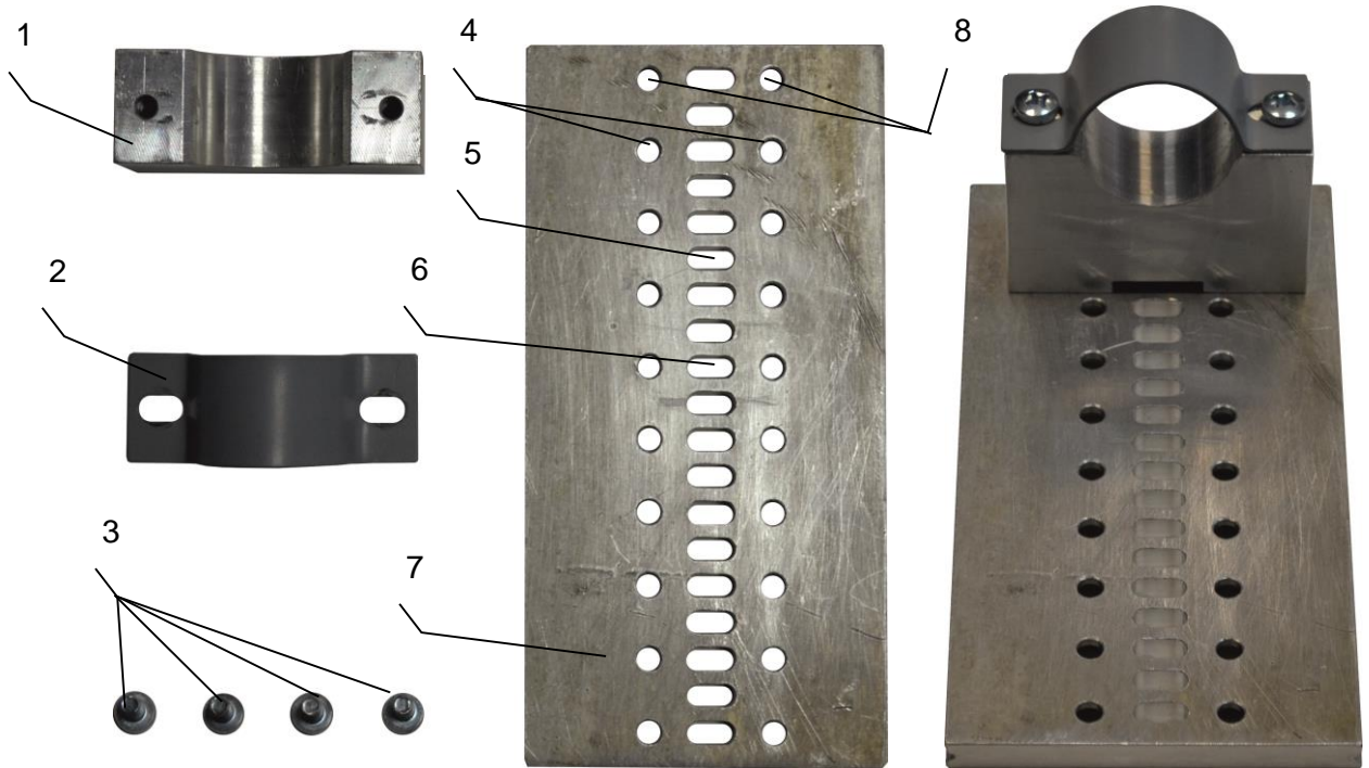
Рисунок 2.2.1.11 – Крепеж облучателя в собранном и разобранном виде.
