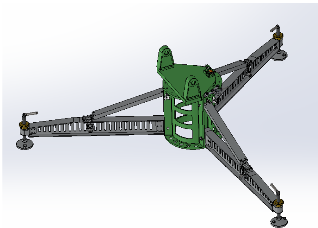
Рисунок 2.2.1.3 – ОПУ и опоры АС
