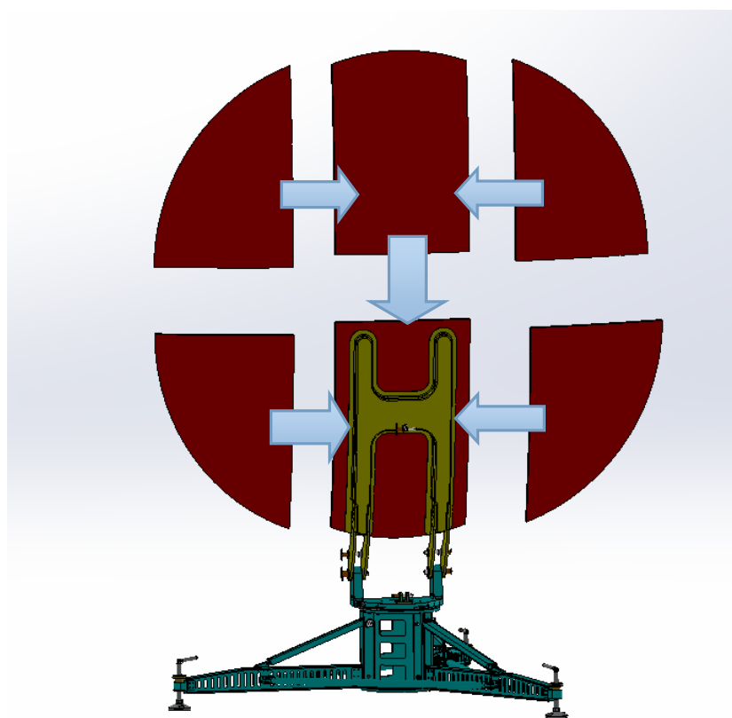
Рисунок 2.2.1.8 – Установка лепестков рефлектора
