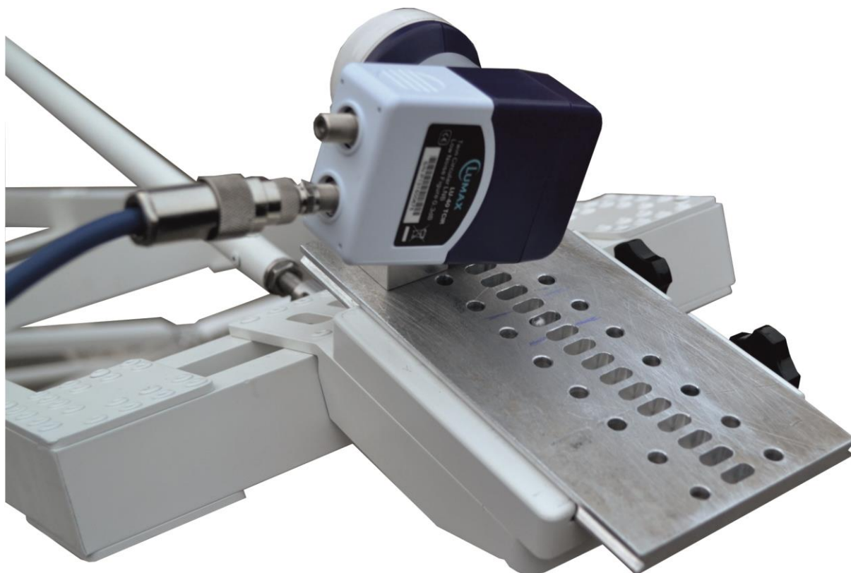
Рисунок 2.2.1.13 – Установка облучателя модели LU-40 TCIR
