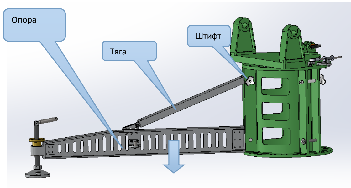
Рисунок 2.2.1.2 – Установка первой опоры АС
