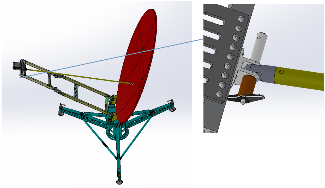
Рисунок 2.2.1.10 – Установка растяжки
