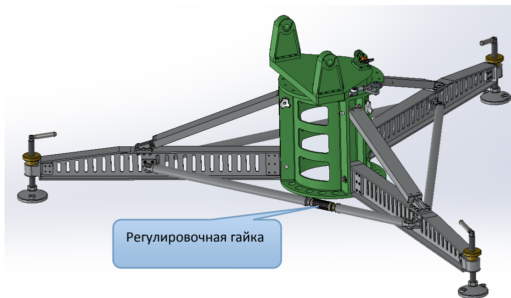
Рисунок 2.2.1.5 – Установка регулировочной тяги
