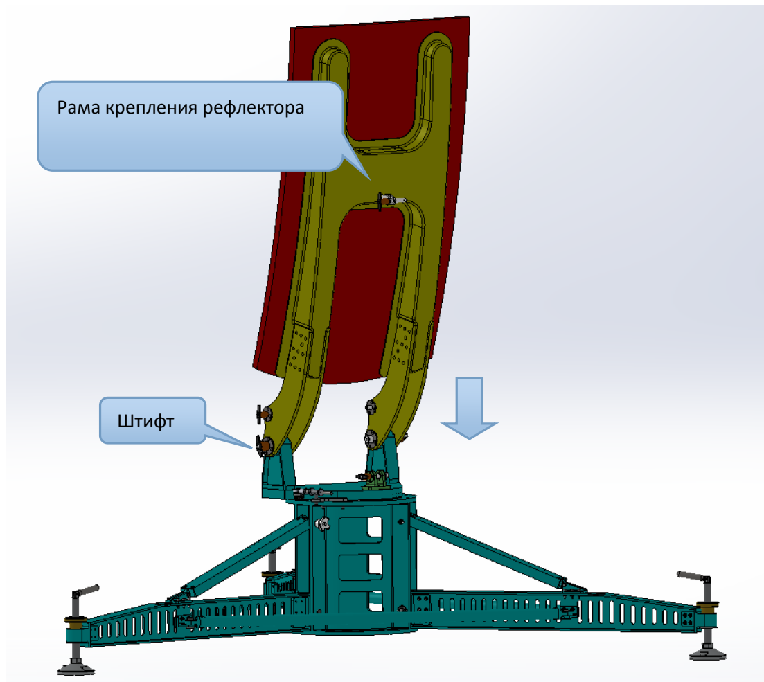
Рисунок 2.2.1.6 – Рама крепления рефлектора
