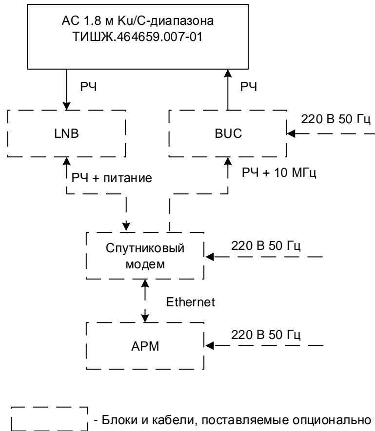
Рисунок 1.1.4 - Функциональная схема АС 1.8 м Ku/C-диапазона
