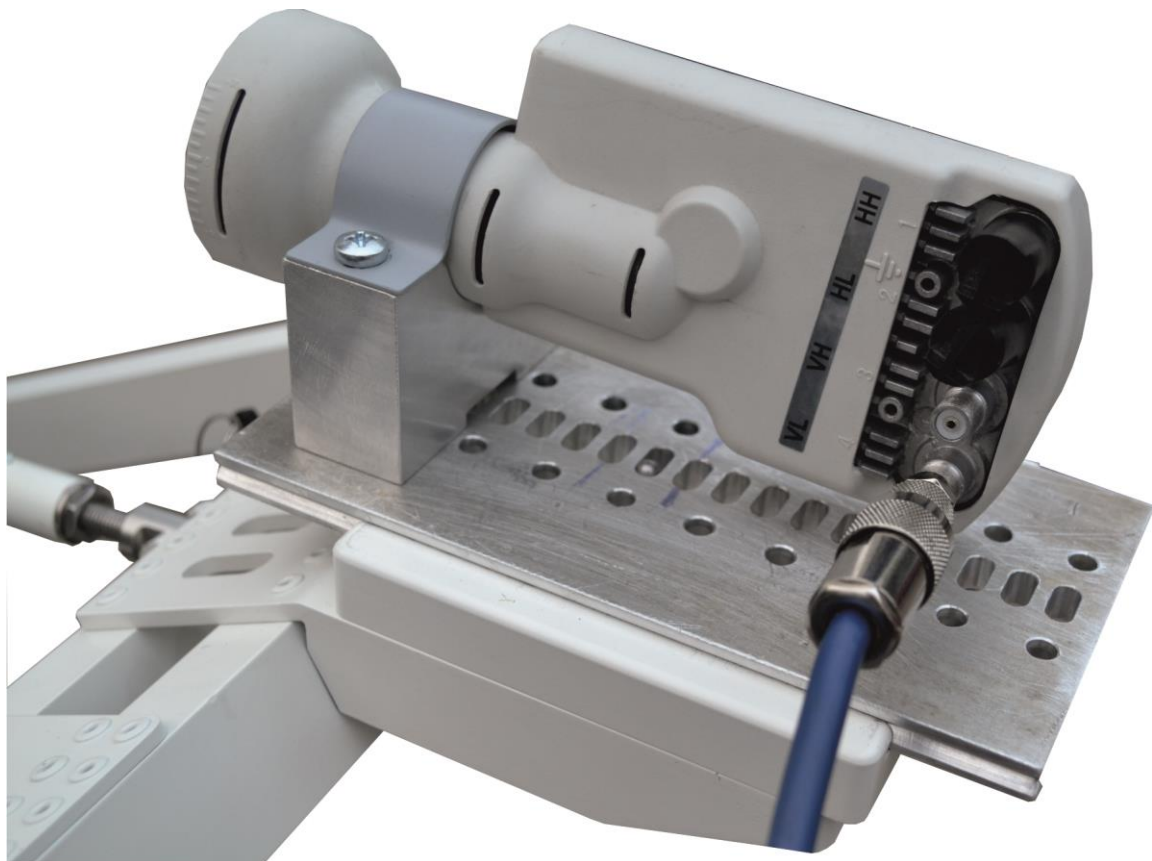
Рисунок 2.2.1.14 – Установка облучателя модели QTH-031
