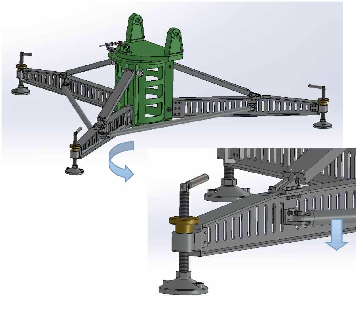
Рисунок 2.2.1.4 – Установка фиксирующих тяг
