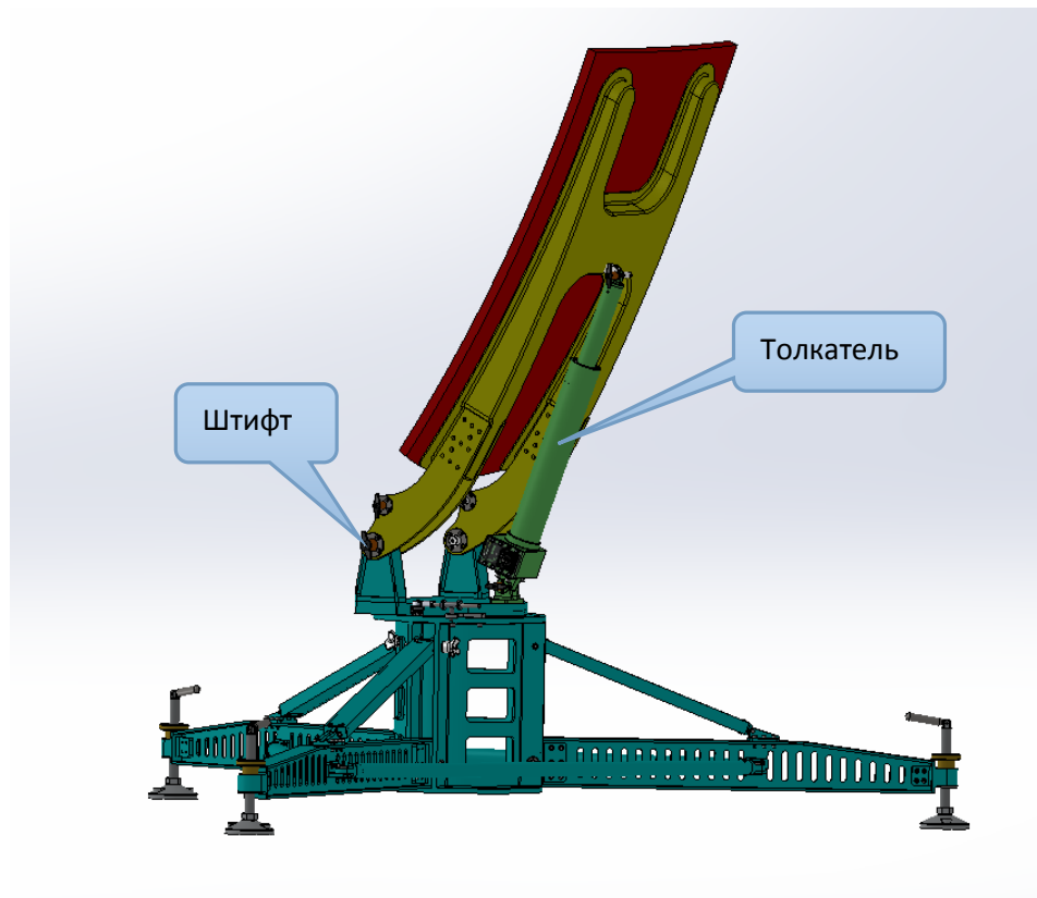
Рисунок 2.2.1.7 – Установка толкателя
