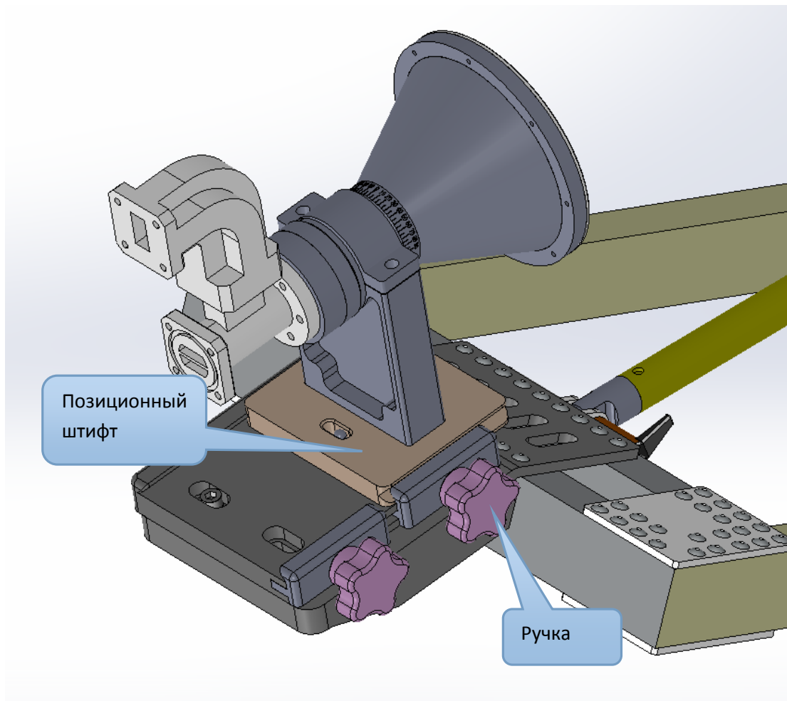
Рисунок 2.2.1.12 – Установка приемопередающего облучателя
